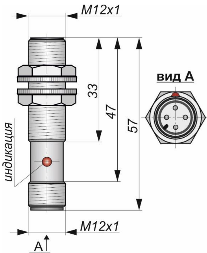
Габаритный чертеж
