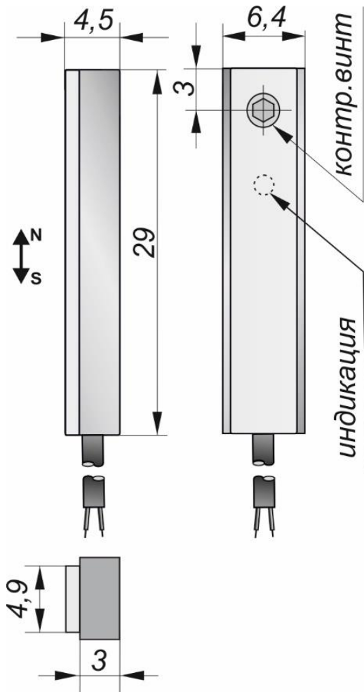
Габаритный чертеж
